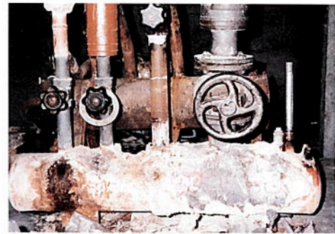
Λέβητες, καυστήρες στο σχολείο Tsanko Tserkovski, Βουλγαρία 1998
